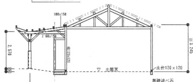
a 通り架橋図 1/100
