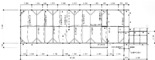
駅舎平面図 1/100
