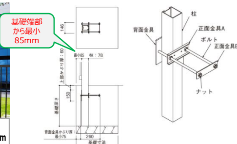
T280(自立建て納まり)上・中・下 ルシアスフェンスH07型 (T100×3)
